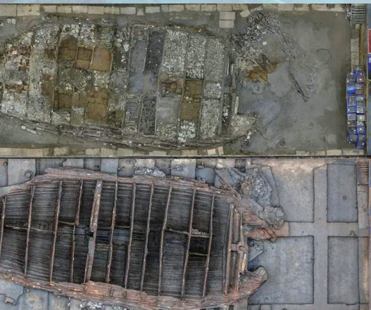
2019 年船货清理完成再后期处理去掉支护沉箱和船体的钢梁、钢管后的正摄影像。
