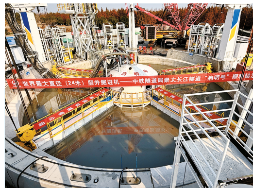
“启明号”投入崇太长江隧道2号竖井建设 采访对象 提供
