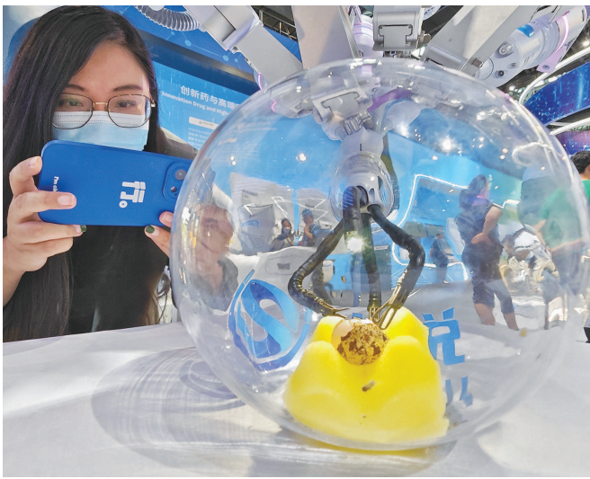
▲ 机器人“茶艺师”的蓝色“夹爪”能模拟煮茶师倒水、泡茶、倒茶等一系列动作 ▲ 单孔腔镜手术机器人系统的镍钛合金蛇形手术臂展示剥鹌鹑蛋的蛋壳
