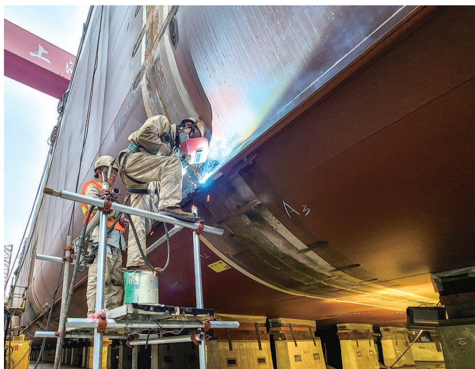
● 昨天,在上海外高桥造船有限公司的船坞内,工人正对我国首艘大型邮轮船底部分进行焊接作业,目前邮轮项已转入连续搭载新阶段 本报记者 陈梦泽 摄
