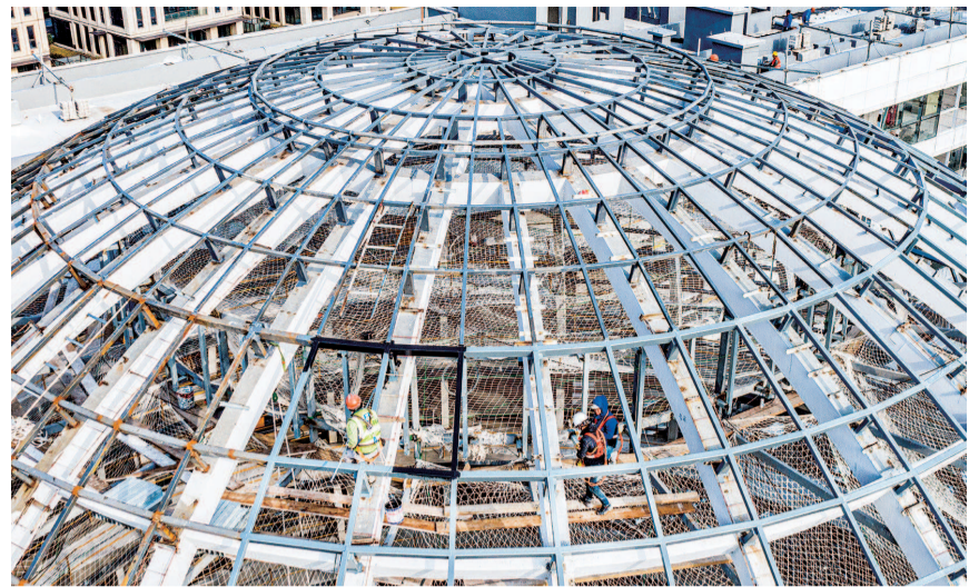
● 昨天,张江科学城内,工人正在李政道研究所上进行幕墙及室内装饰工程。李政道研究所作为上海科创中心建设重点任务和张江综合性国家科学中心的重要组成部分,将在量子与核物理、天文与天体物理、量子基础科学三个方向开展重大科学问题研究 本报记者 孙中钦 摄
